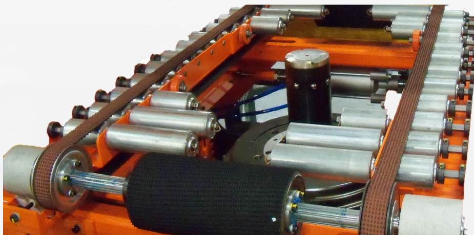
AIT上的皮带和辊筒
